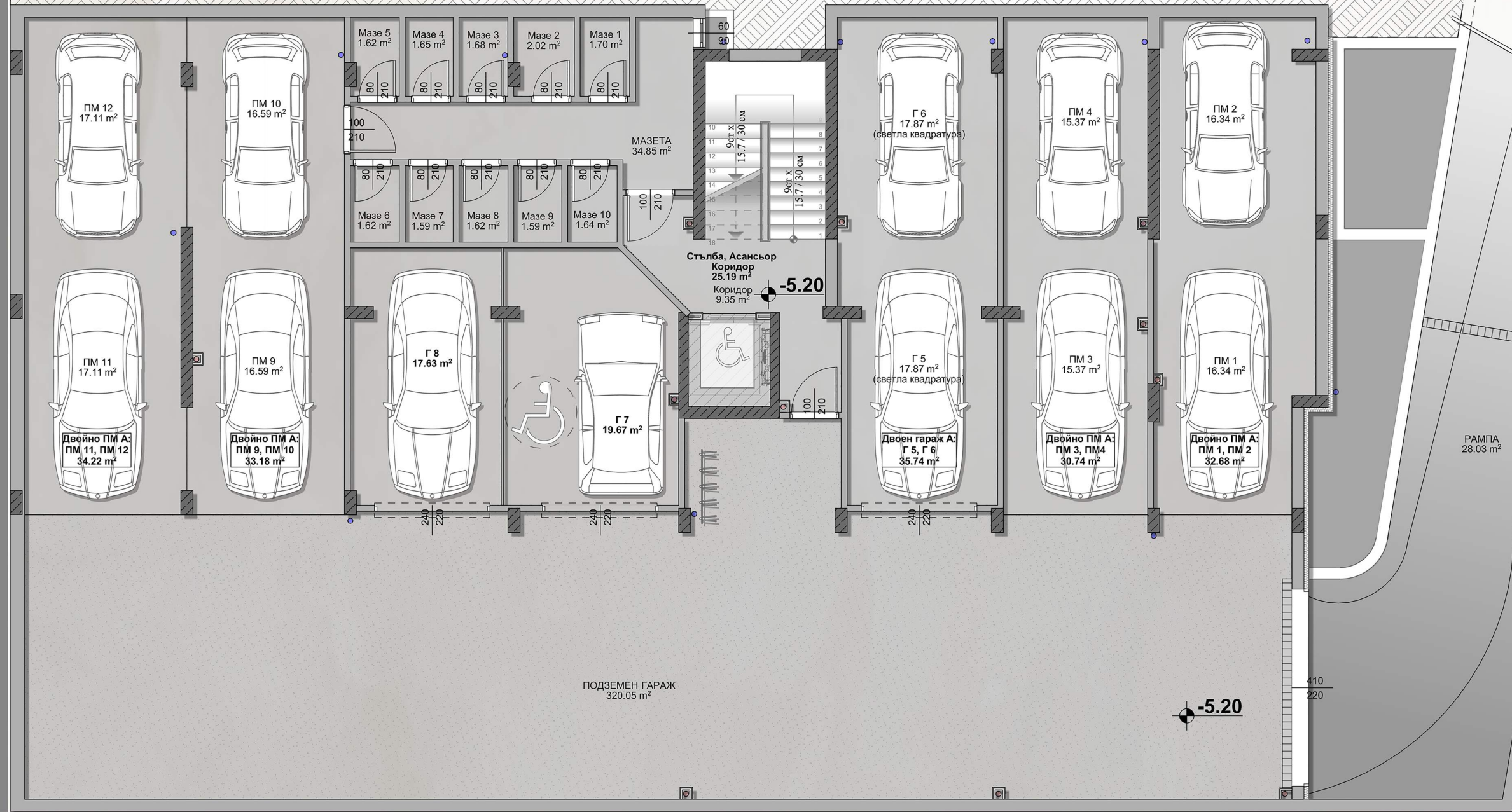
Сграда А, Сутерен -2, Кота - 5,20
